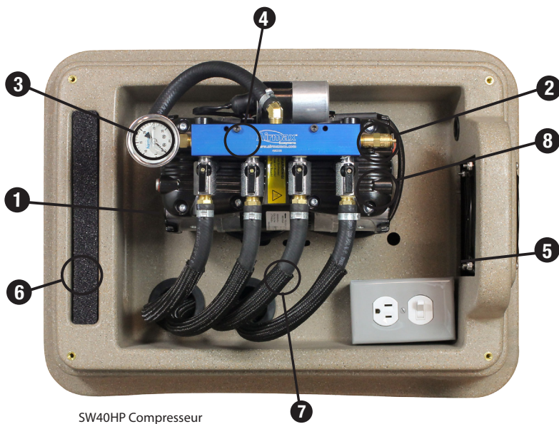
SW40HP Compresseur
